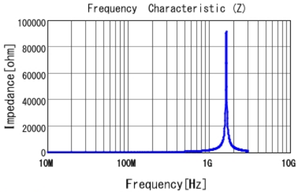
LQW18ANR18J00 |Z|
