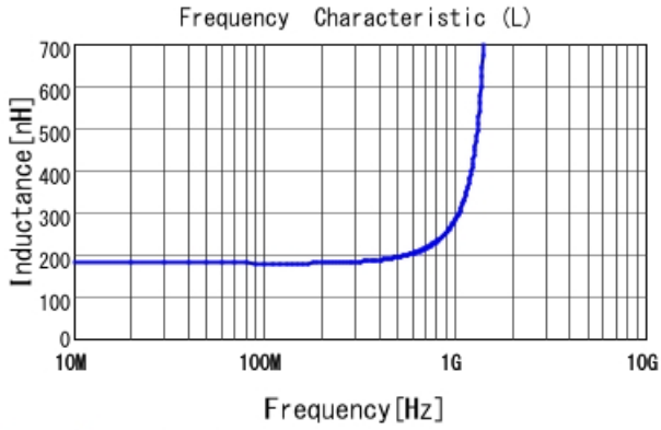
LQW18ANR18J00 L
