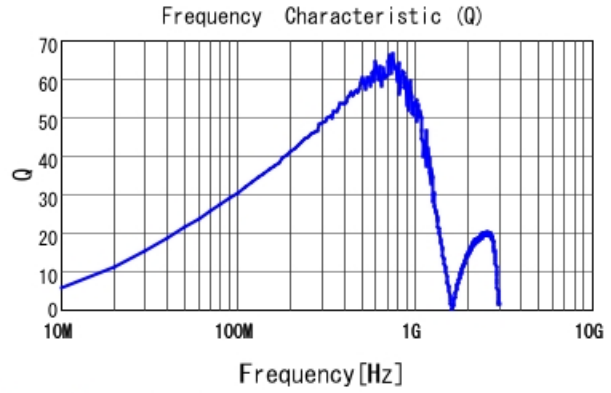
LQW18ANR18J00 Q
